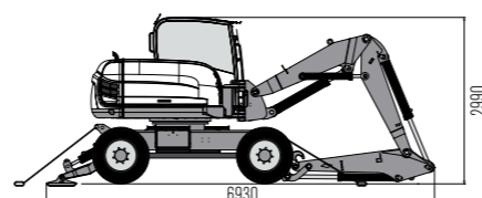
Abb. 3: Transportstellung
